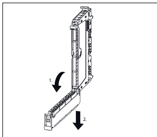
Anschlussrahmen öffnen und Steckverbinderereinheit abziehen
