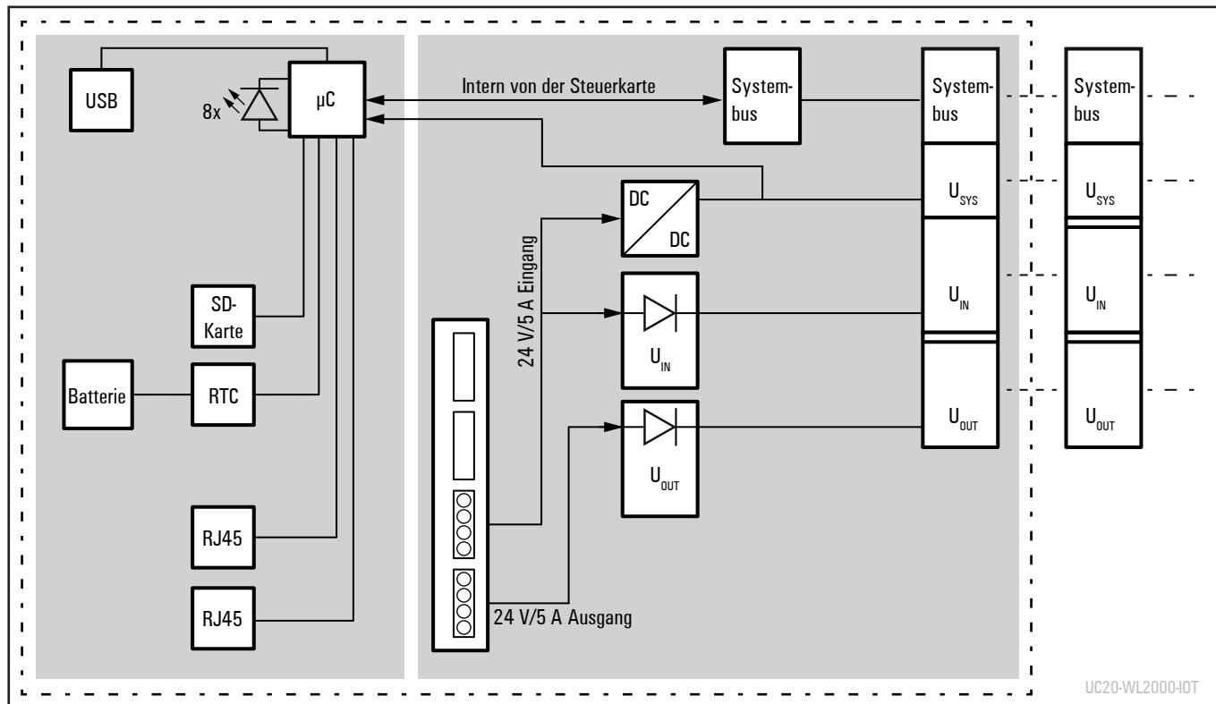
Blockschaltbild UC20-WL2000-IOT
