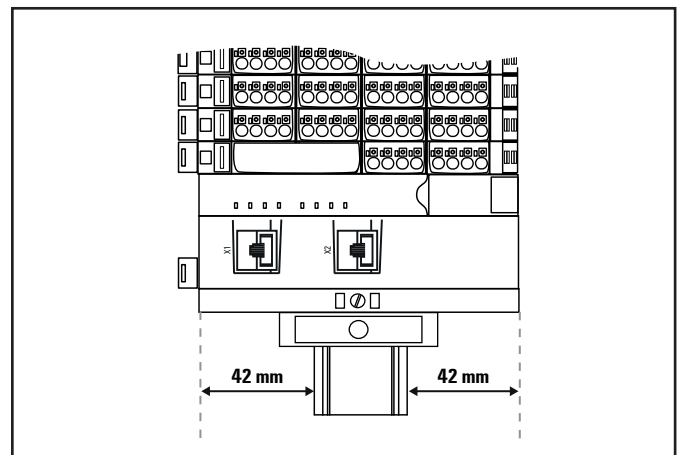
Einbauweise u-control-Station auf Tragschiene (vertikale Montage)
