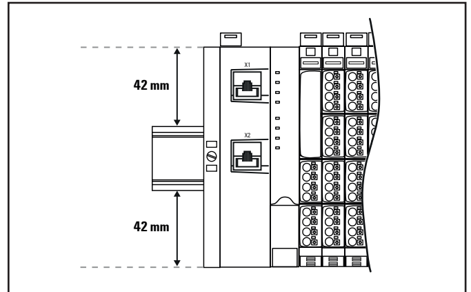
Einbauweise u-control-Station auf Tragschiene (horizontale Montage)
